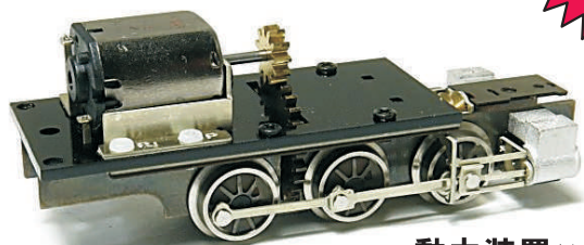
動力装置(組立済)
